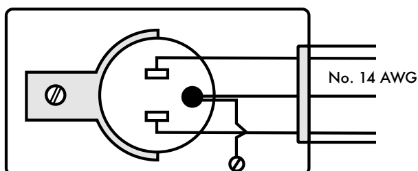
Toma tripolar con conexión a tierra
