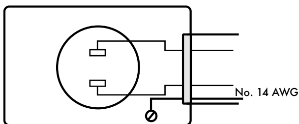
Toma bipolar con conexión a tierra
